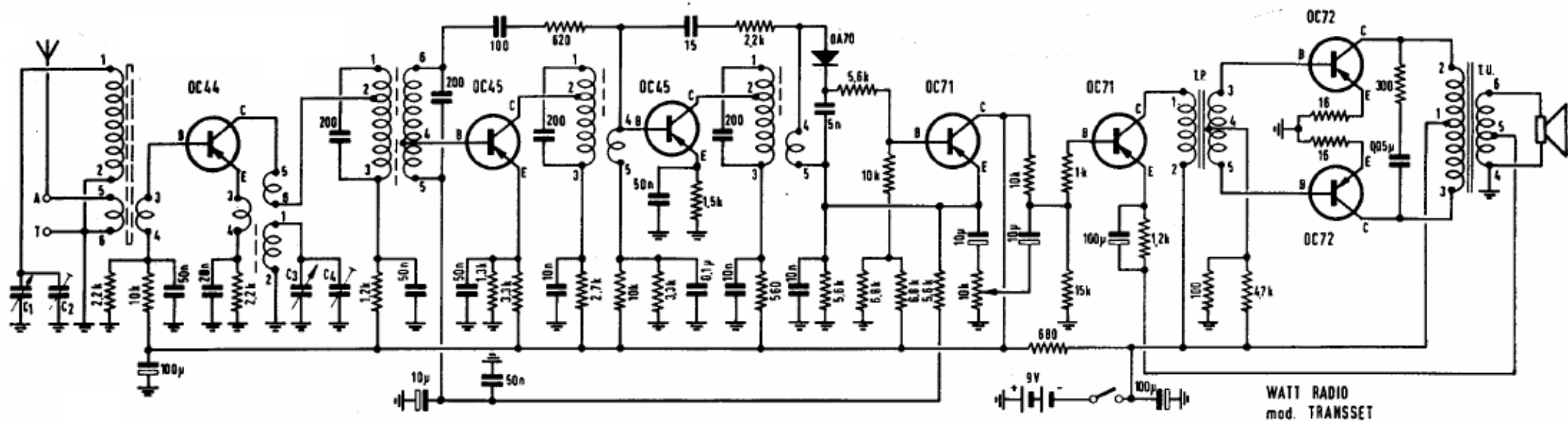
Schema elettrico del radoricevitore Watt Radio, mod. TRANSSET
